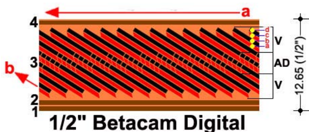
Figura 138. Estructura de pistas Betacam Digital
