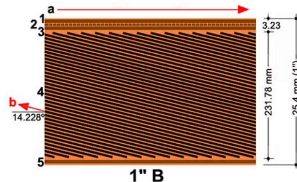
Figura 133. Estructura de pistas Formato 1 pulgada B
