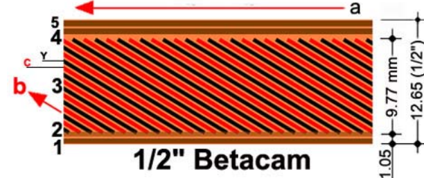
Figura 137. Estructura de pistas Formato Betacam
