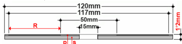
Figura 61. Dimensiones estandarizadas para discos de lectura óptica laser.
