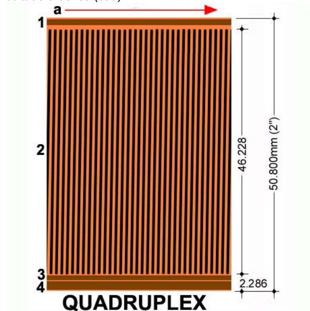
Figura 130. Estructura de pistas formato Quadruplex
