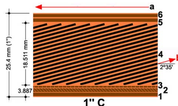
Figura 134. Estructura de pistas Formato 1 pulgada C
