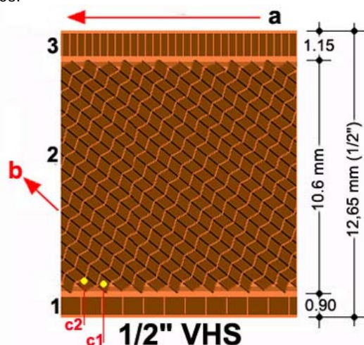
Figura 136. Estructura de pistas Formato VHS
